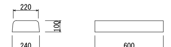
乗入れ部 10cm (32kg)
