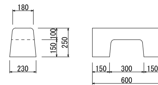
水抜き部 (53kg)
