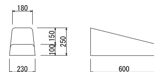
切下げ部10cm (51kg)
