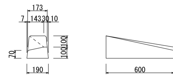
切下げ部 (36kg)
