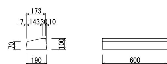
乗入れ部 (25kg)
