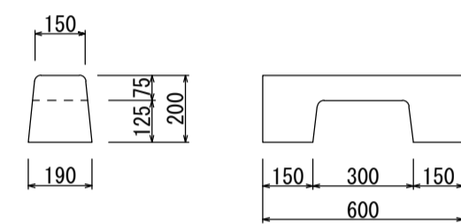
水抜き部 (32kg)
