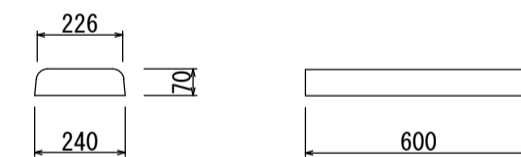
乗入れ部 7cm (23kg)
