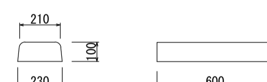
乗入れ部 10cm (30kg)
