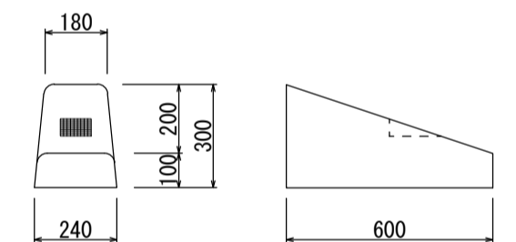
切下げ部(反射板付) 10cm (60kg)
