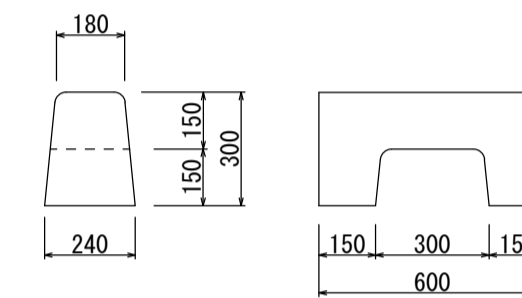
水抜き部 (65kg)
