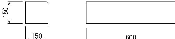
地先C（面取り）（31kg）
