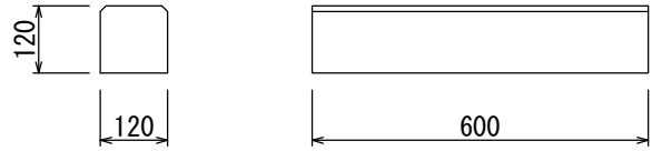
地先A（両面取り）（20kg）
