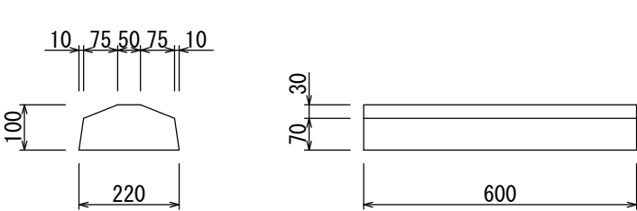
水止ブロック（26kg）
