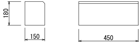
並木樹ブロック 3号（29kg）
