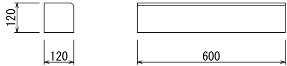
地先A（面取り）（20kg）
