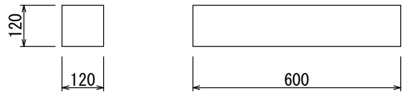
地先A（面無し）（20kg）
