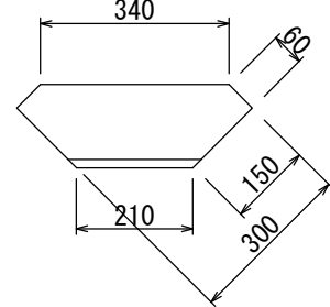
並木樹ブロック 5号（21kg）
