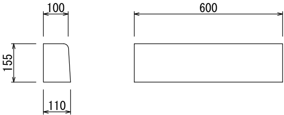
公園ブロック（24kg）
