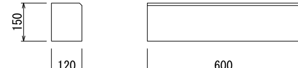
地先B（面取り）（25kg）
