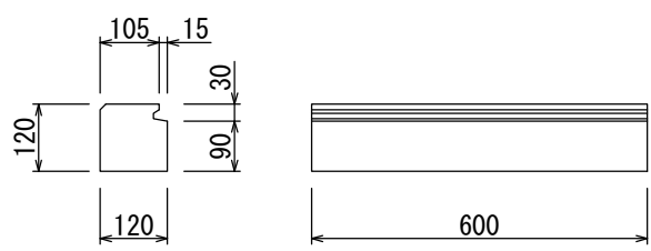
地先A（面取り・草防止仕様）（19kg）
