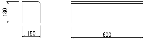
並木樹ブロック 2号（38kg）
